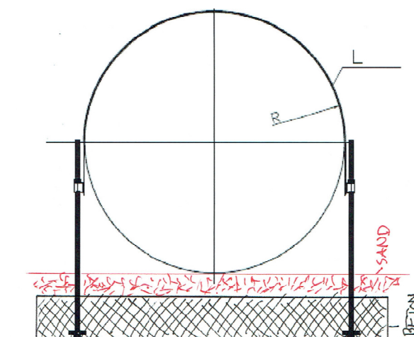
Principskitse med forankringsbånd og ankere
